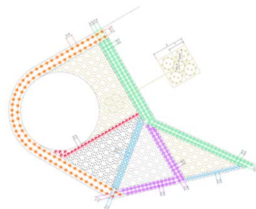
zoom plantación 1 e: 1/100
