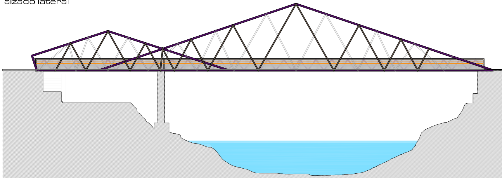
sección transversal
